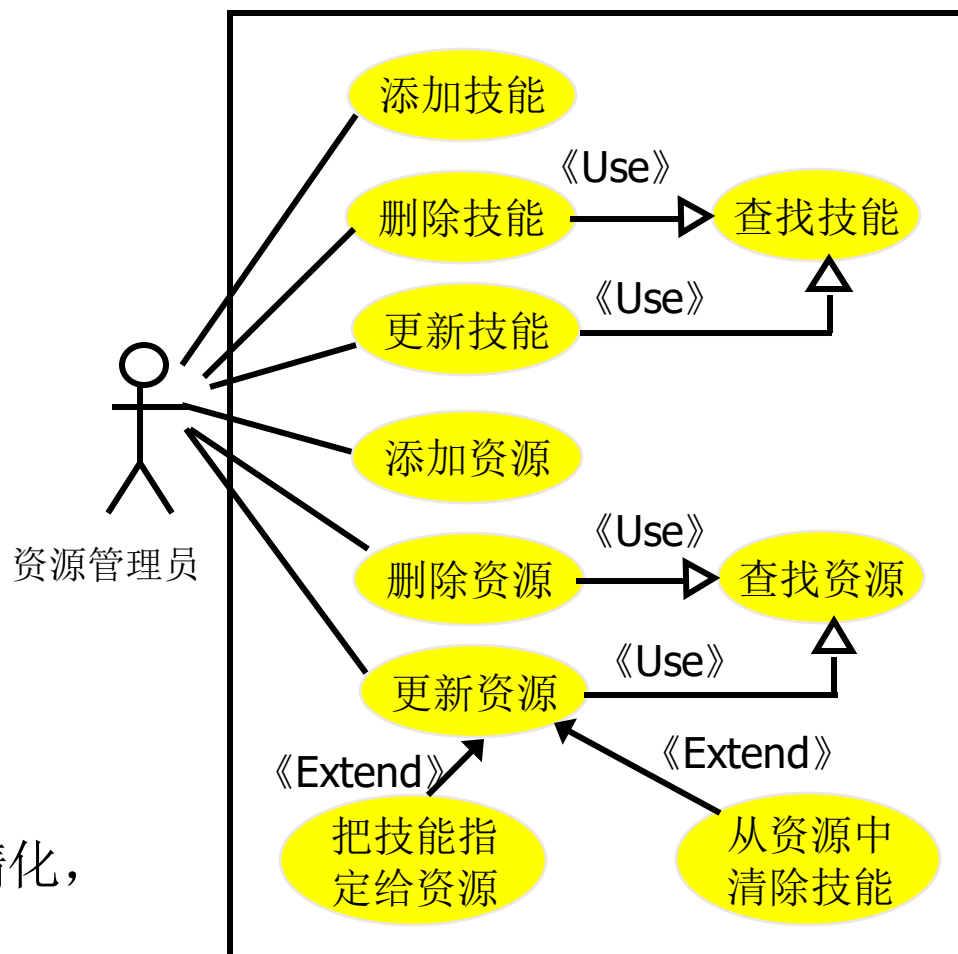
资源管理Use Case图
