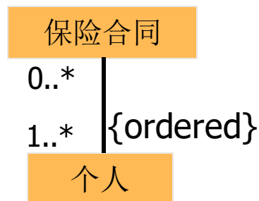
(a)指定链接之间有明确的顺序
