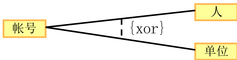
对象类的xor关联
