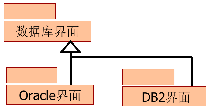
(c) 包的泛化关系
