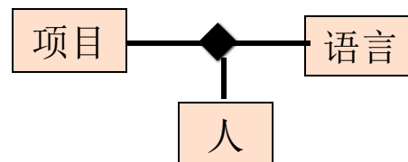
三元关联的例
